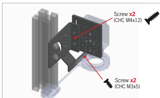
TPL-MOUNT-TRING-V1
