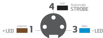
VUE DE FACE DU CONNECTEUR DU PRODUIT
